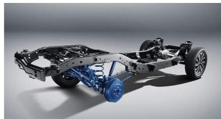
Hệ thống treo sau 5 liên kết
